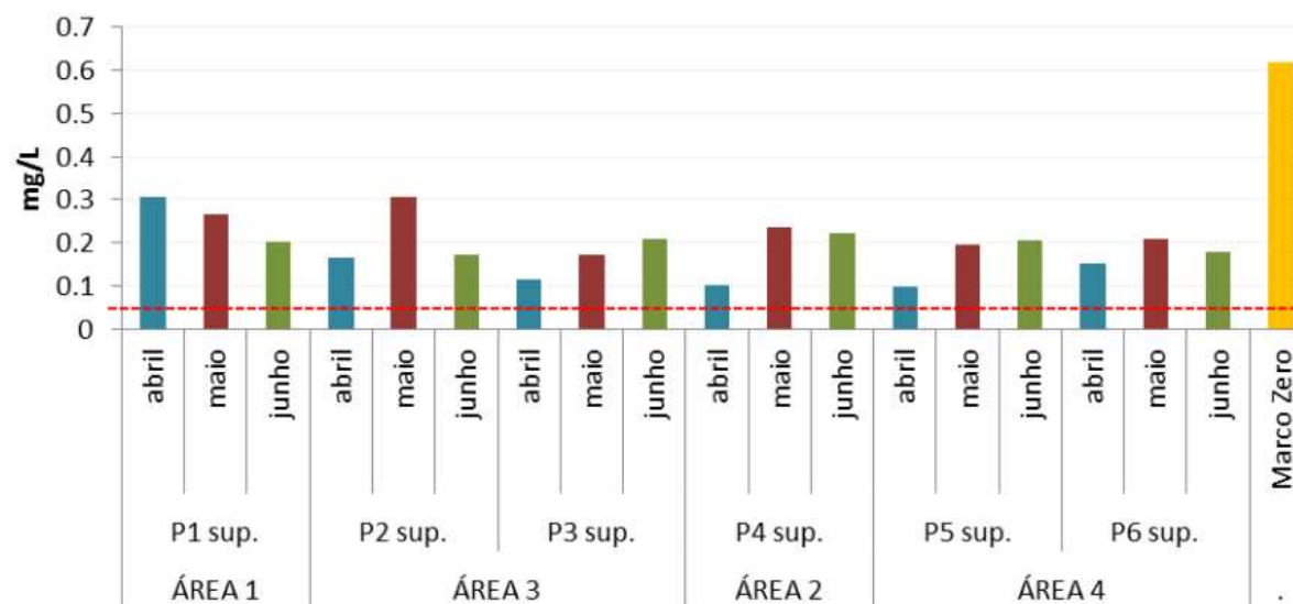
Figura 72 - Concentrações de fósforo total (mg/L) da superfície da Lagoa da Pampulha obtidas em abril, maio e junho de 2016.
