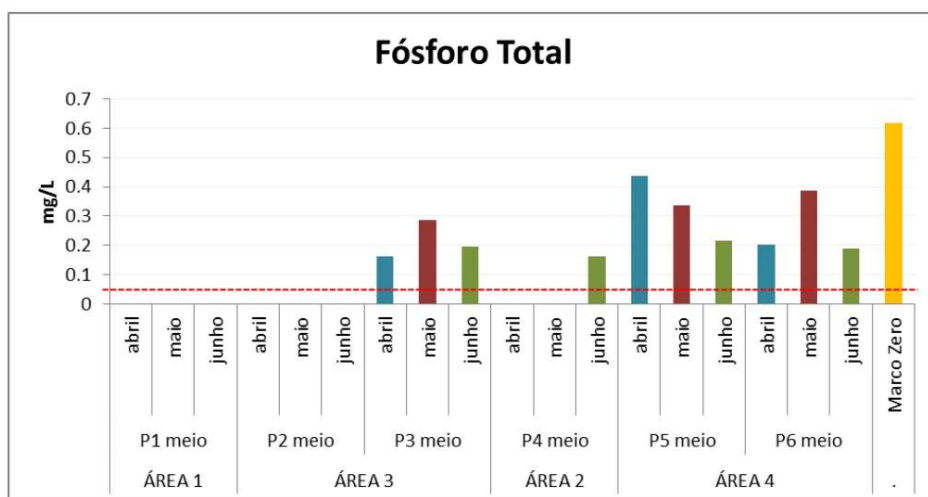
Figura 73 - Concentrações de fósforo total (mg/L) do meio da coluna d'água da Lagoa da Pampulha obtidas em abril, maio e junho de 2016.
