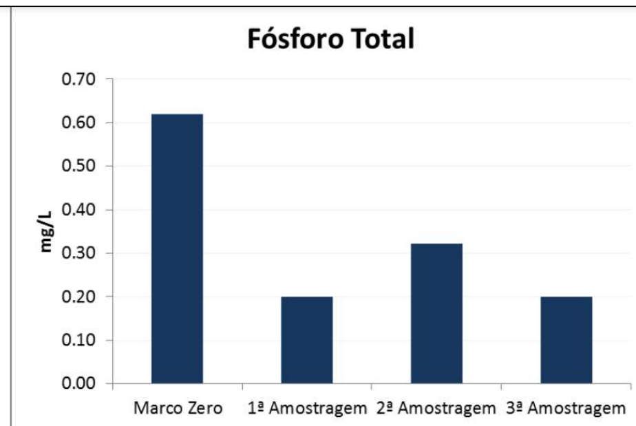
Figura 76 - Concentração de fósforo total de referência para avaliação do tratamento (Marco Zero) e concentrações mensais médias observadas na coluna da água durante evolução do tratamento.
