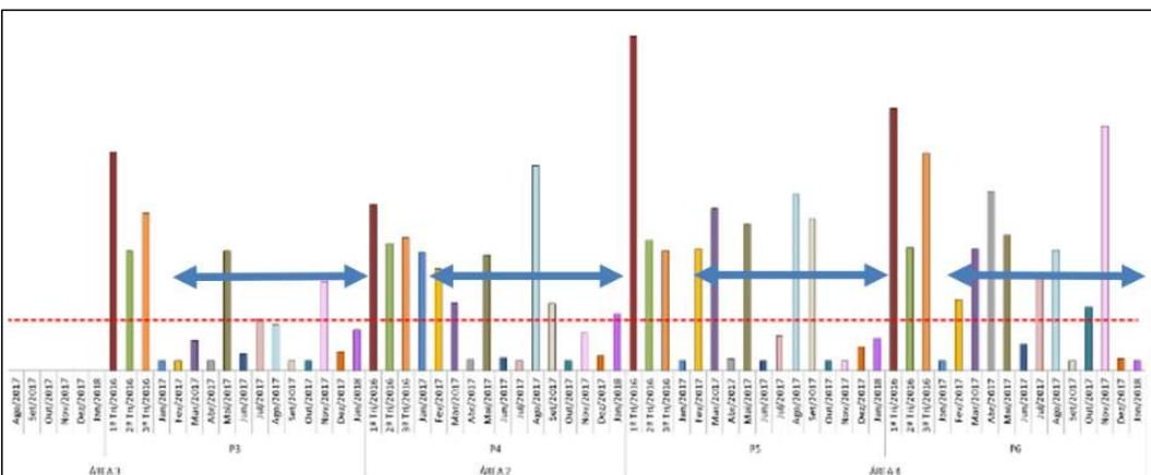
RELATÓRIO TRIMESTRAL – 7º TRIMESTRE, p. 143, Figura 63 – Concentrações de fósforo total (mg/L) do meio da coluna d'água da Lagoa da Pampulha obtidas nos três primeiros trimestres de monitoramento de 2016 (Abril à Dezembro) a Janeiro de 2018.
