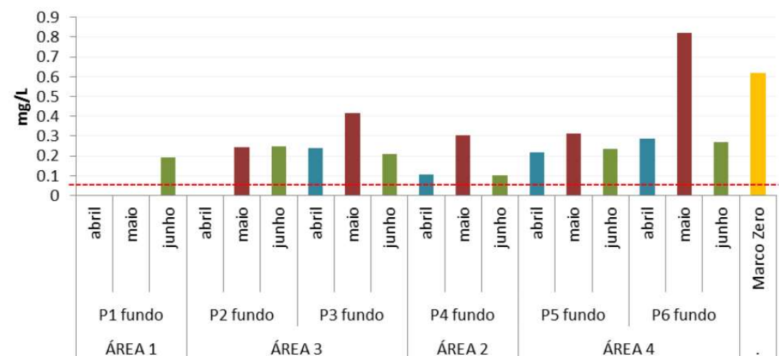
Figura 74 - Concentrações de fósforo total (mg/L) do fundo da coluna d'água da Lagoa da Pampulha obtidas em abril, maio e junho de 2016.
